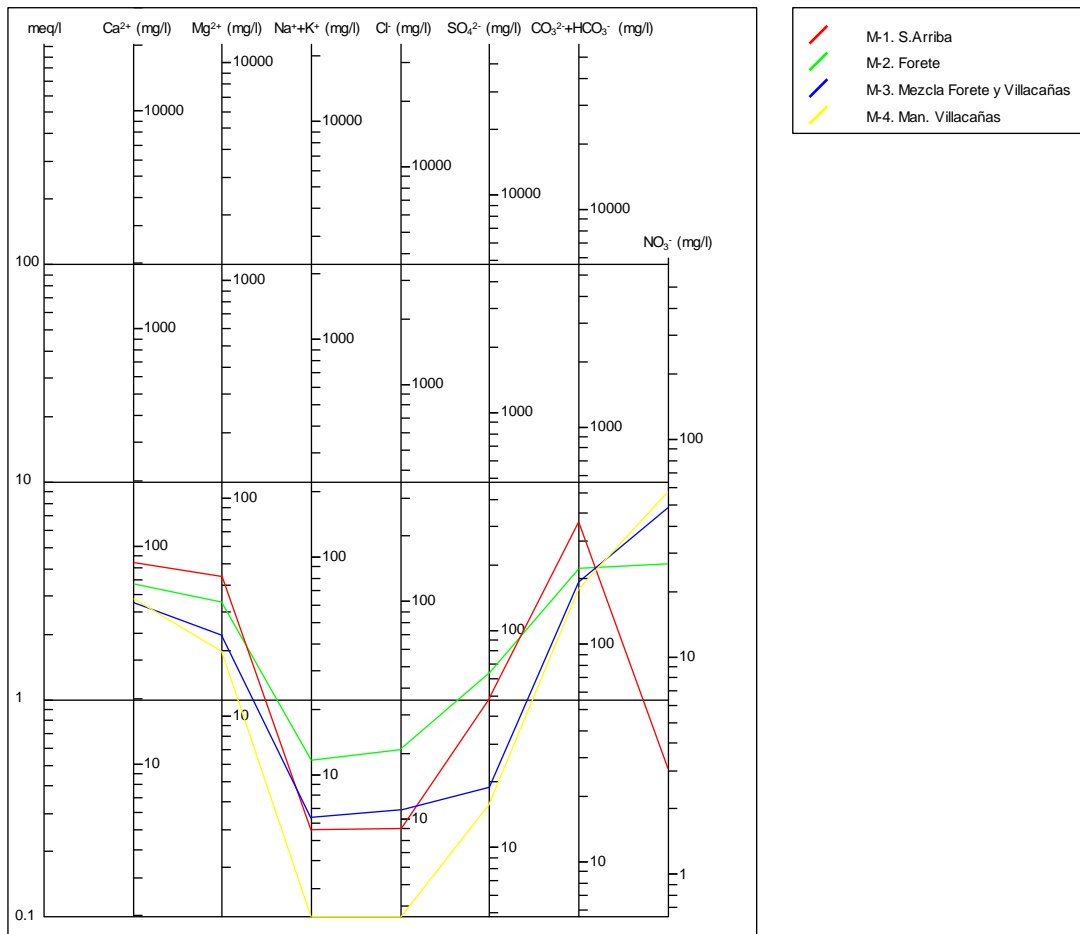
Figura 8. Diagrama de Schöeller de las 4 muestras
