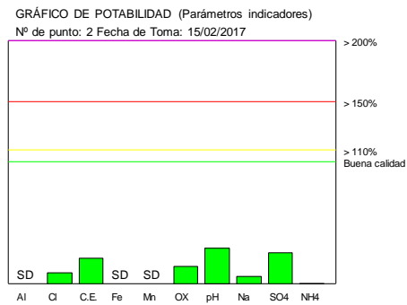
Figura 14. Gráfico de potabilidad del Pozo Forete
