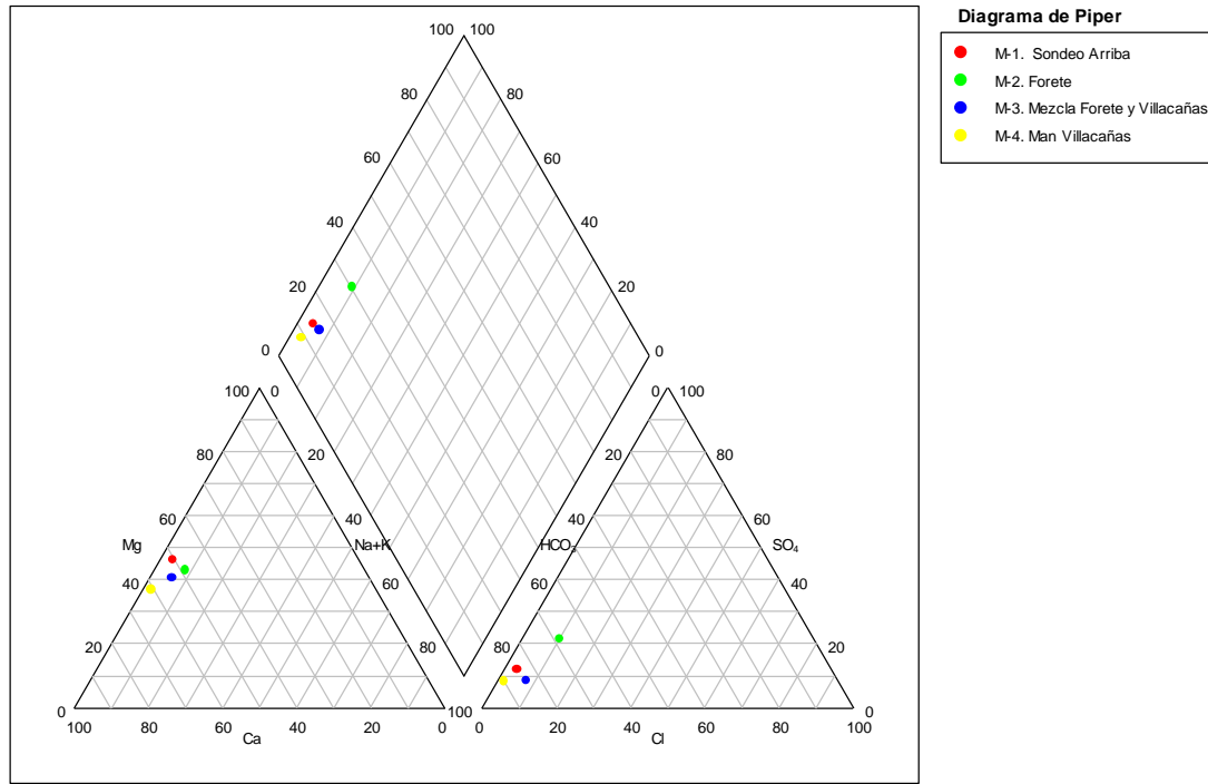
Figura 6. Diagrama de Piper-Hill-Langelier de las 4 muestras
