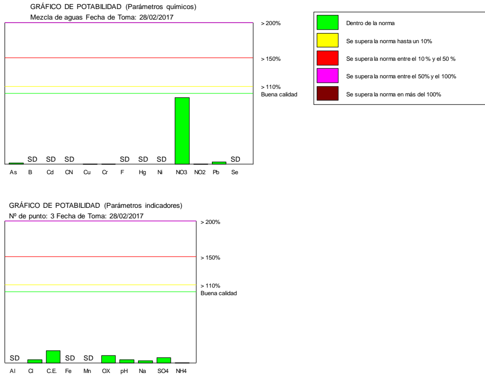
Figura 15. Gráfico de potabilidad de la mezcla de aguas Forete y Villar de Cañas
