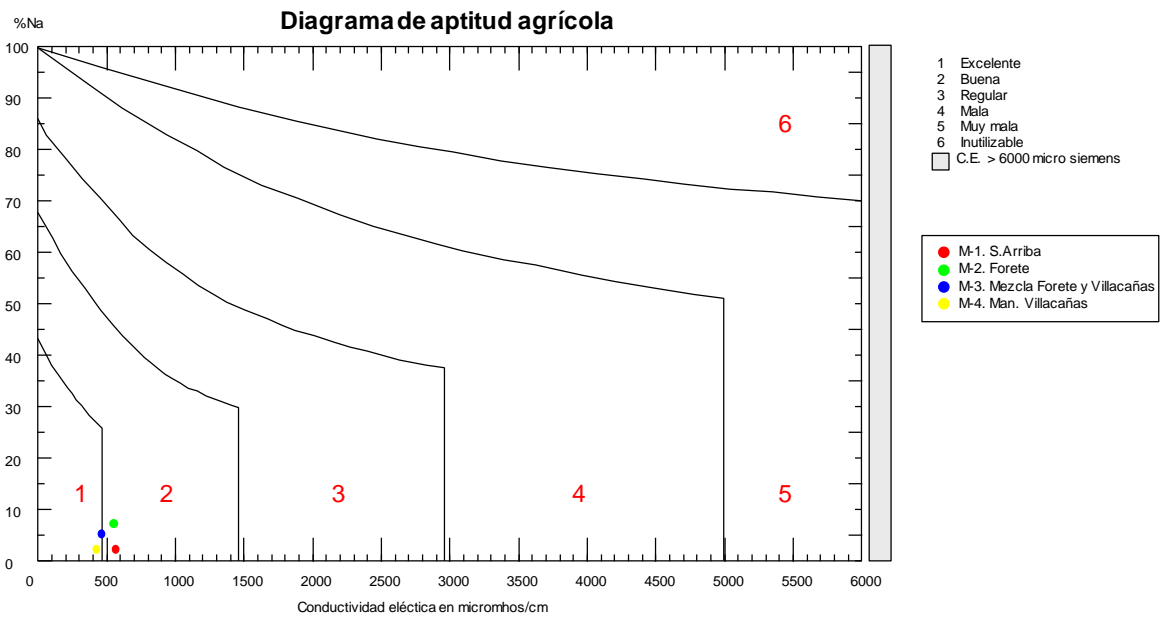
Figura 7. Diagrama de altitud agrícola de las 4 muestras
