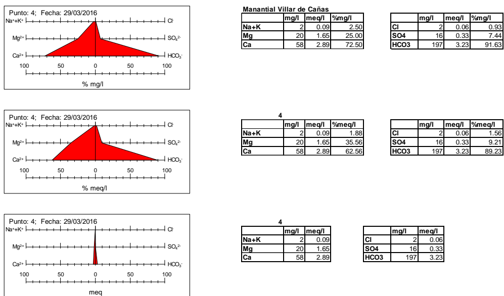
Figura 12. Diagrama de Stiff del manantial Villar de Cañas
