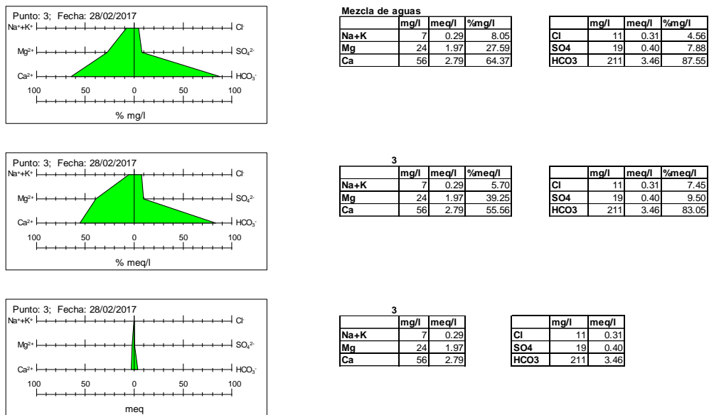
Figura 11. Diagrama de Stiff de la mezcla de aguas Forete y Villar de Cañas
